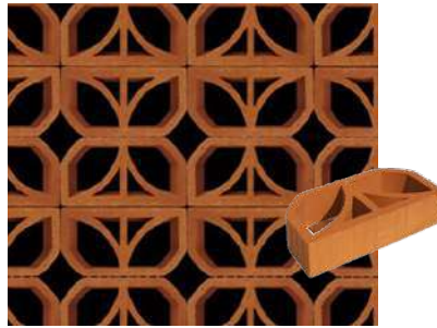
Celosía N° 3 1.5kg/pza 32 pzas/m 2 • 24x12x6cm
