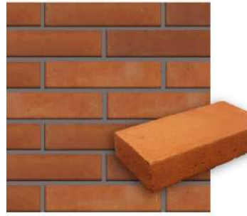
Tabique Rojo Recocido 2VR 24x12x6cm 57 pzas/m 2 • 1.8kg/pza
