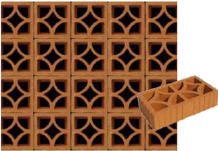
Celosía N° 1 1.8kg/pza 30 pzas/m 2 • 24x13x6cm
