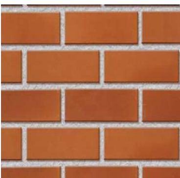
Cintilla de Barro 2VC 23x6x2cm 57 pzas/m 2 • .4kg/pza
