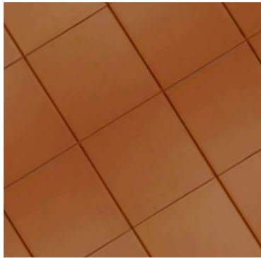
Loseta de Barro 16 pzas/m 2 • 24x24x2cm
